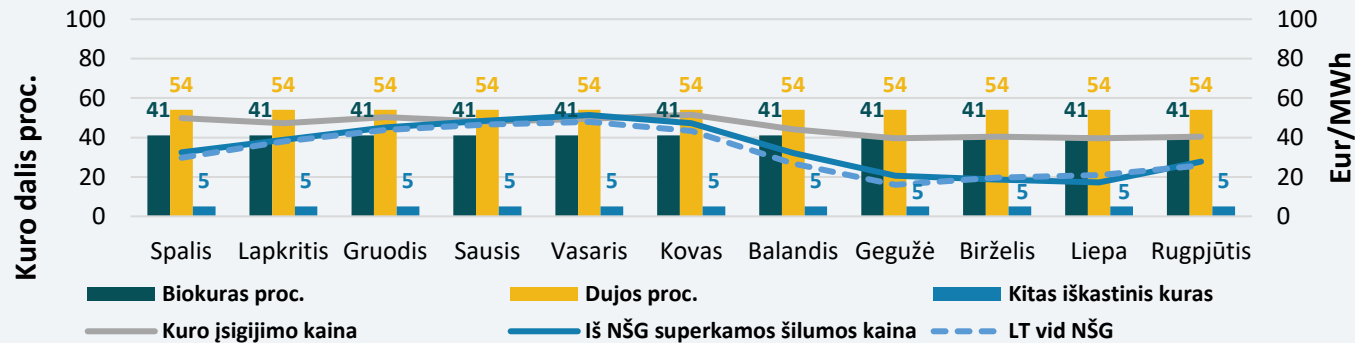
Šilumos tiekėjo nuosavos gamybos kuro struktūra ir superkamos iš NŠG* šilumos kaina Kaune (2024–2025 m.)
