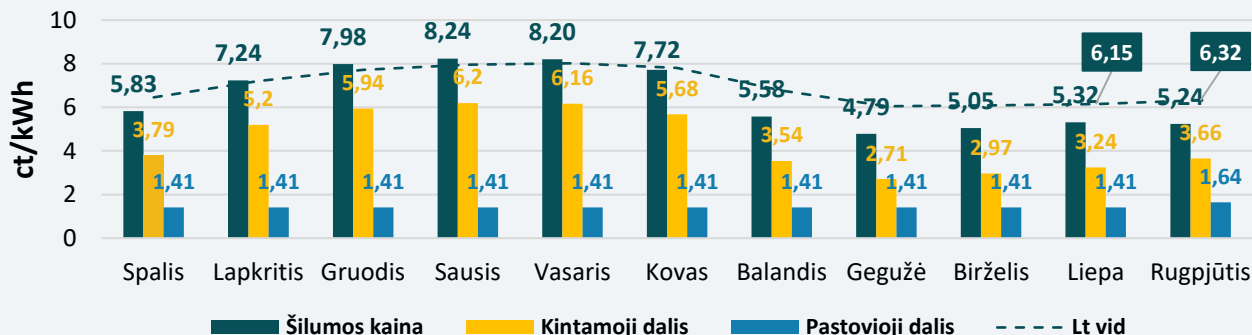
Šilumos energijos kainos struktūra (be PVM) Vilniuje (2024–2025 m.)
